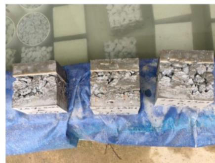
Gambar 4. Hasil Sampel Persentase Superplasticizer 2% Dan Terdapat Rongga.
