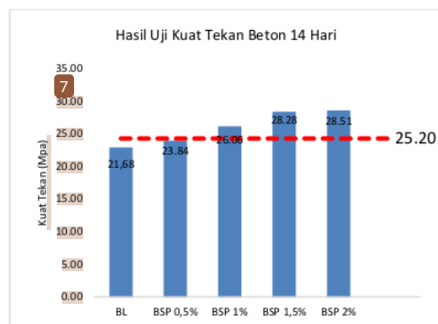
Gambar 2. Perbandingan Nilai Kuat Tekan Pada Umur 14 Hari
