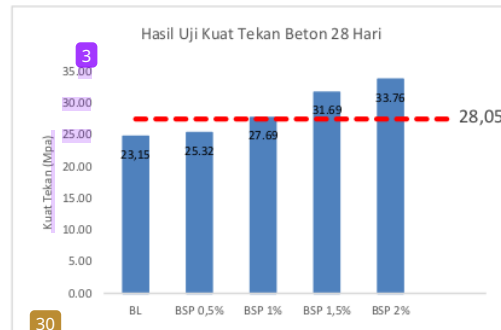
Gambar 3. Perbandingan Nilai Kuat Tekan Pada Umur 28 Hari
