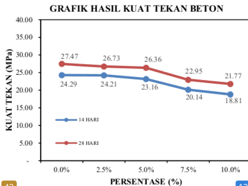
42 Gambar 3. Grafik Kuat Tekan Beton 14 Hari dan 28 Hari 12
