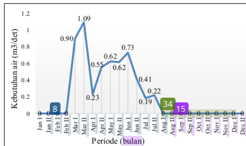
Gambar 3 Grafik Kebutuhan Air
