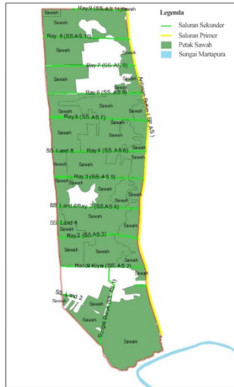
Gambar 1. Skema Jaringan DIR Antasan Sutun
