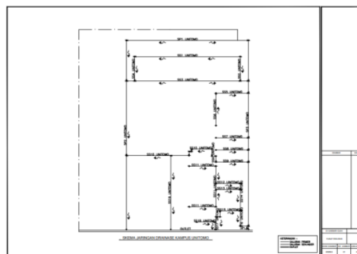
Gambar 4. Skema Jaringan Drainase Rencana
