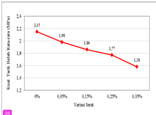
Gambar 4. Grafik Kuat Tarik Belah Beton Terhadap Variasi Serat Pada Umur 28 Hari
