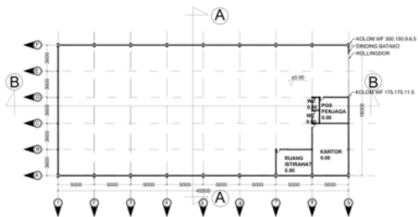
Gambar 2. Denah Bangunan Baja
