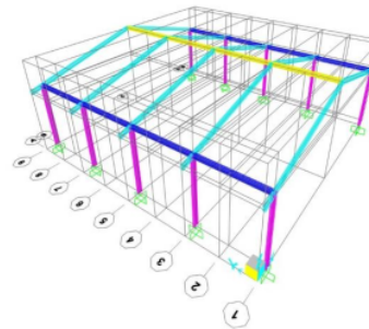
Gambar 4. Pemodelan struktur menggunakan SAP2000
