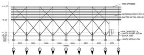
Gambar 3. Gambar Potongan
