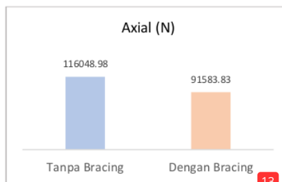
Gambar 5. Perbandingan nilai axial struktur bangunan baja tanpa bracing dan dengan bracing
