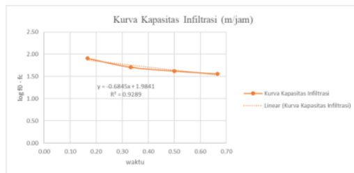
Gambar 3. kurva kapasitas infiltrasi gradien m
