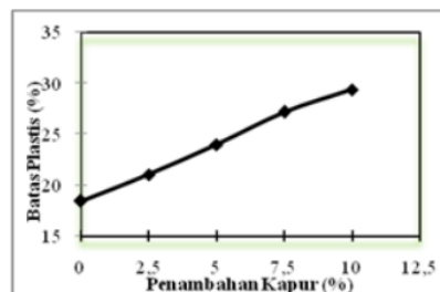
Gambar 3. Variasi Penambahan Kapur Terhadap Batas Plastis
