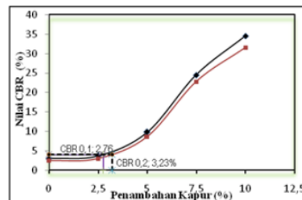
Gambar 9. Batas Minimum Penambahan Kapur untuk CBR=4 .
