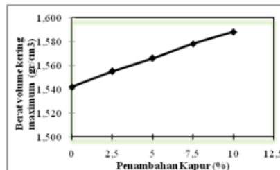
Gambar 5. Variasi Penambahan Kapur Terhadap Harga \gamma_{dmax}
