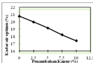
Gambar 6. Variasi Penambahan Kapur Terhadap Kadar air optimum
