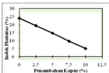
Gambar 4. Variasi Penambahan Kapur terhadap Indeks Plastisitas
