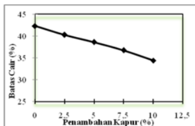
Gambar 2. Variasi Penambahan Kapur Terhadap Batas Cair
