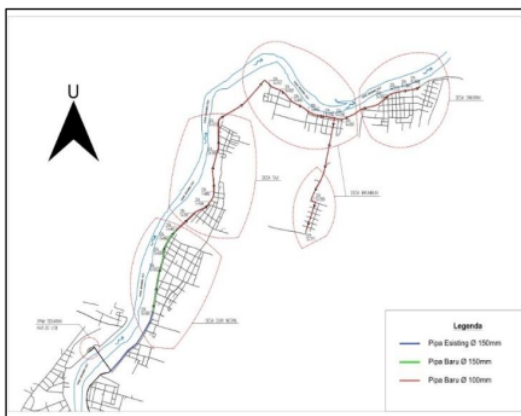
Gambar 4. Pola Sistem Distribusi Hasil Perencanaan
