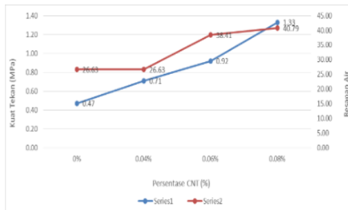
Gambar 7. Kuat Tekan vs Resapan Air
