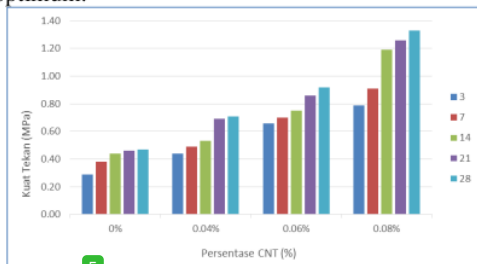
Gambar 5. Kuat Tekan Rata-Rata
