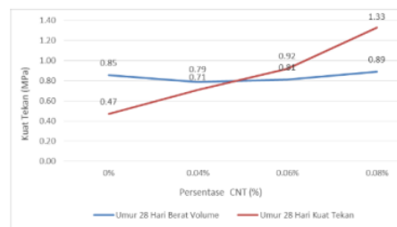
Gambar 6. Berat Volume vs Kuat Tekan
