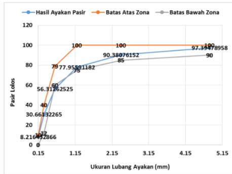
Gambar 1. Gradasi pasir
