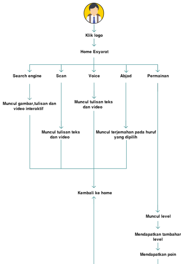
Gambar 5 Interaction Maps Aplikasi E-SYARAT
