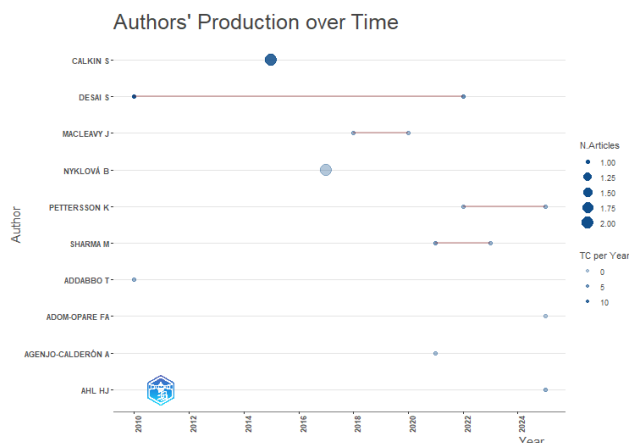
Gambar 2. Produktivitas Penulis
