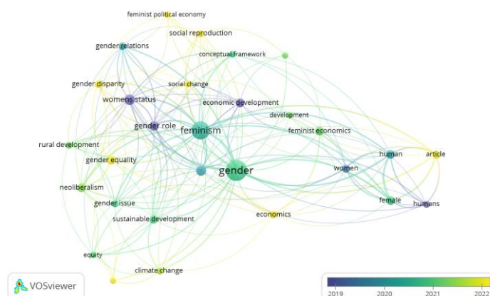
Gambar 5. Visualisasi VOSviewer
